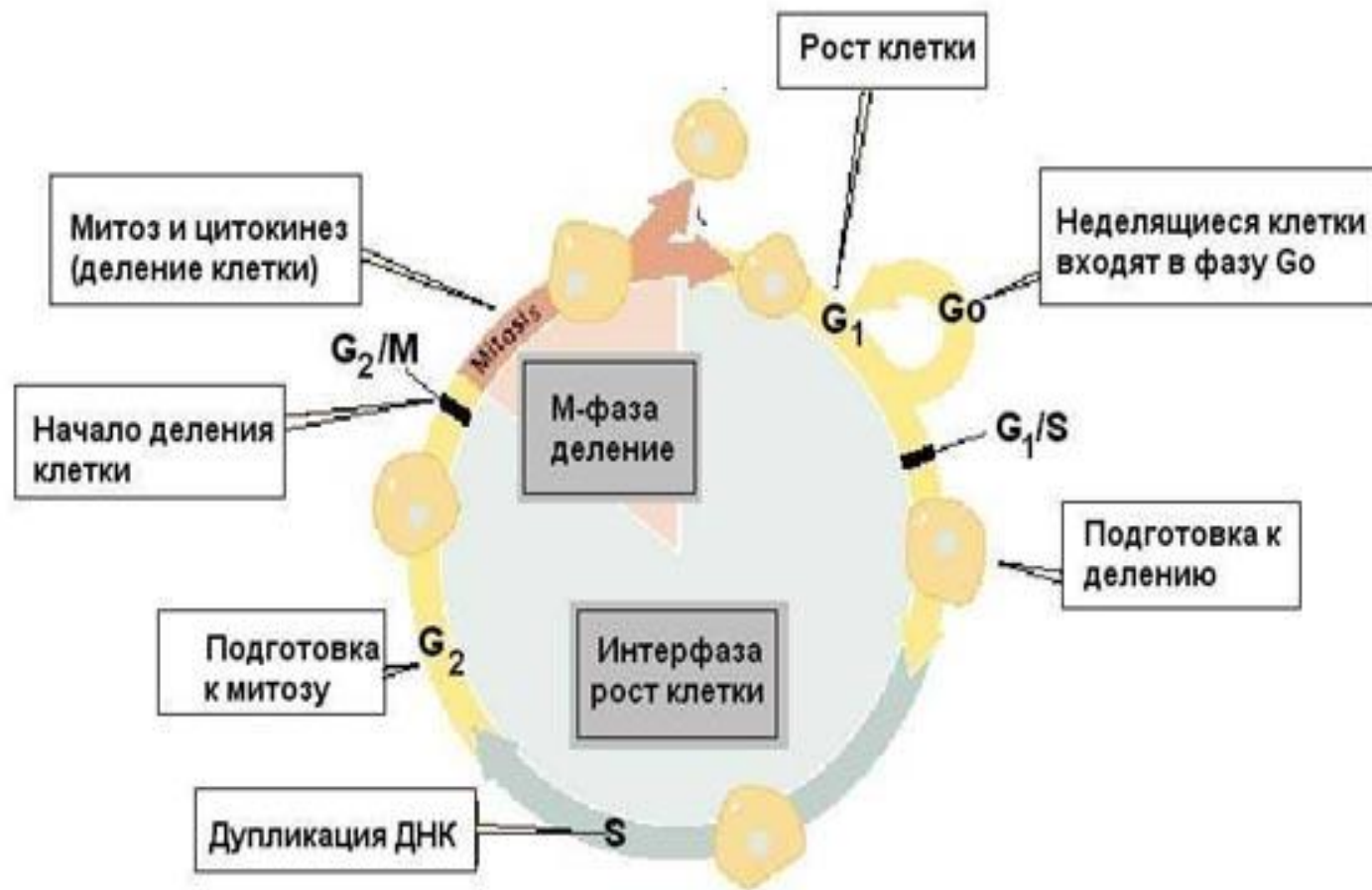
Клеточный цикл
